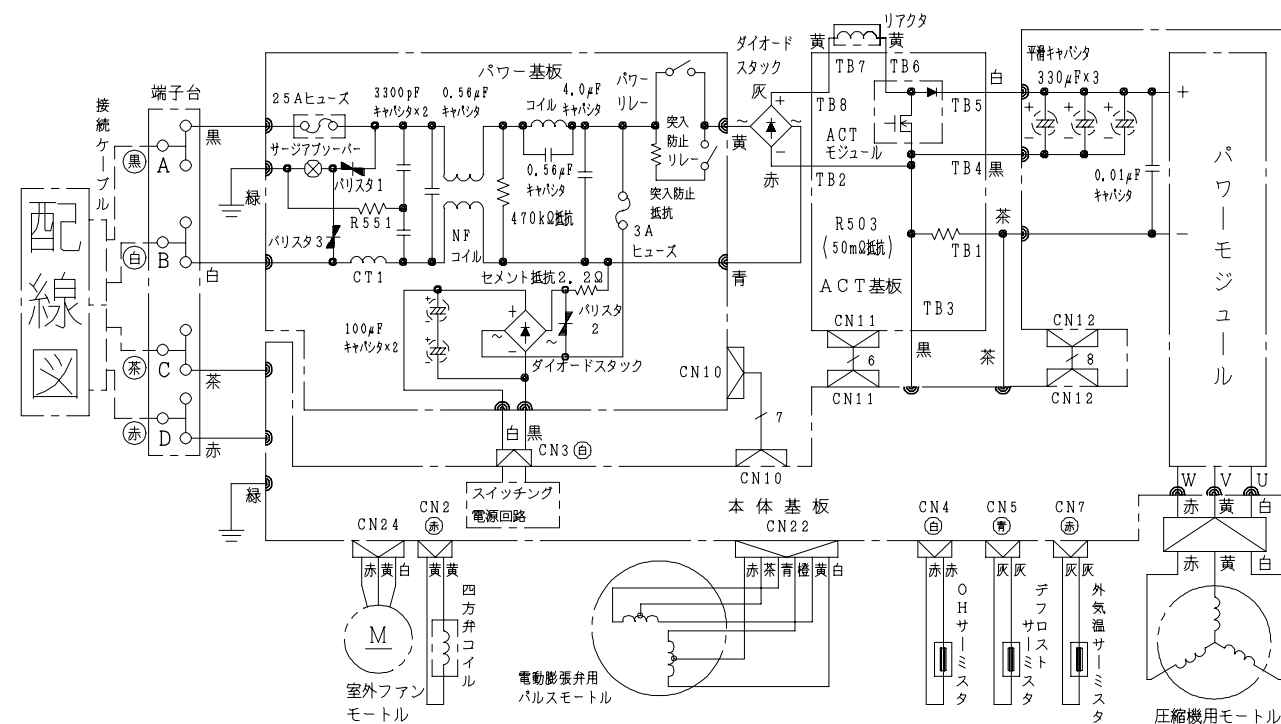
配線図 RAC-4010JX2
