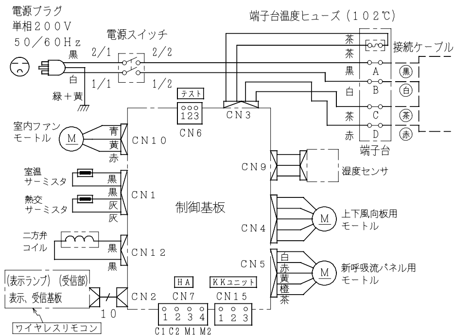
配線図 RAS-4010JX2
