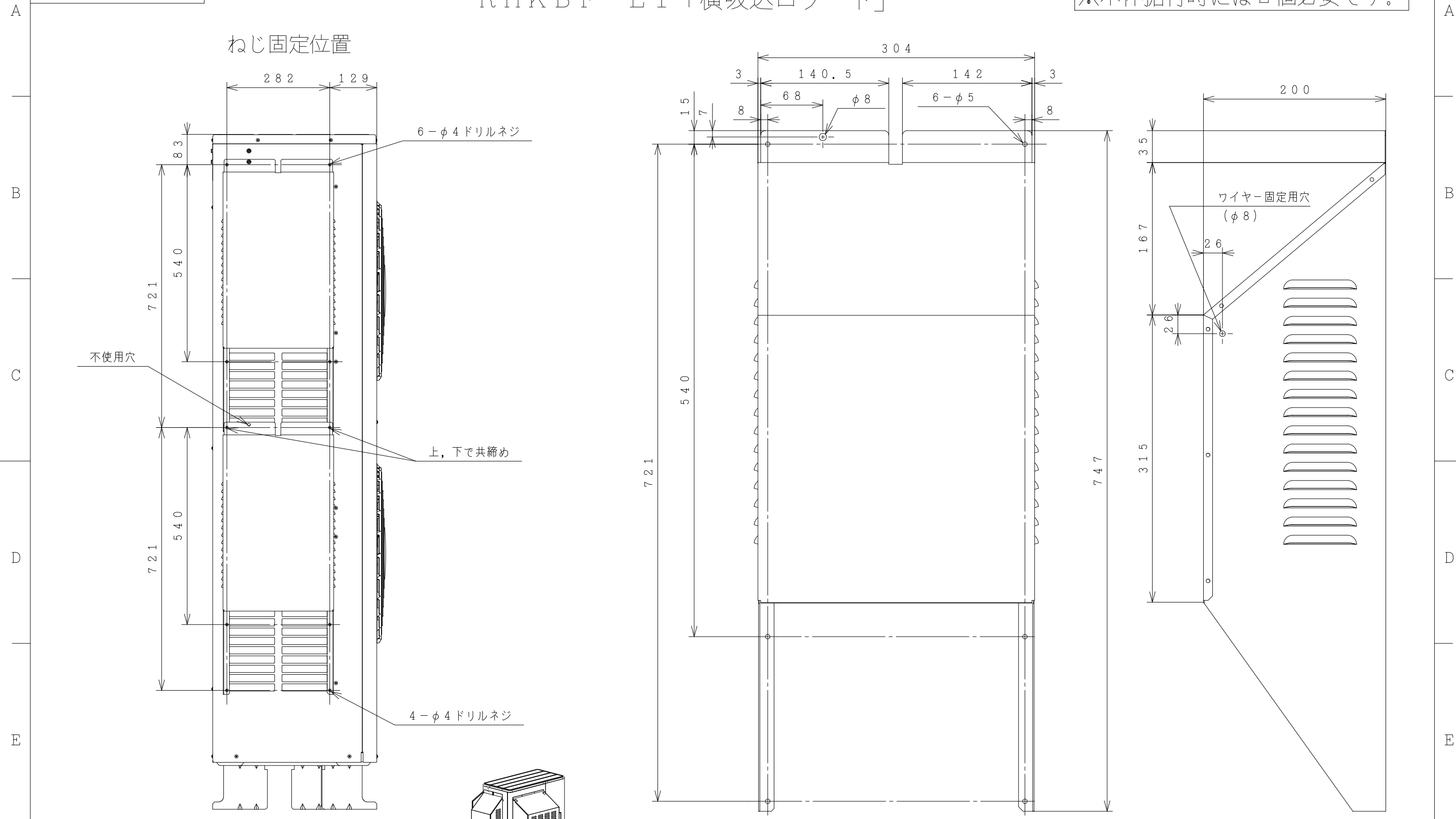
横吸込ロフード
