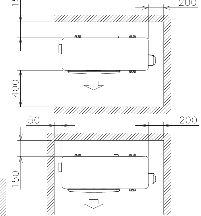
室外機標準据付寸法図
