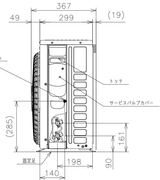
室外機標準据付寸法図
