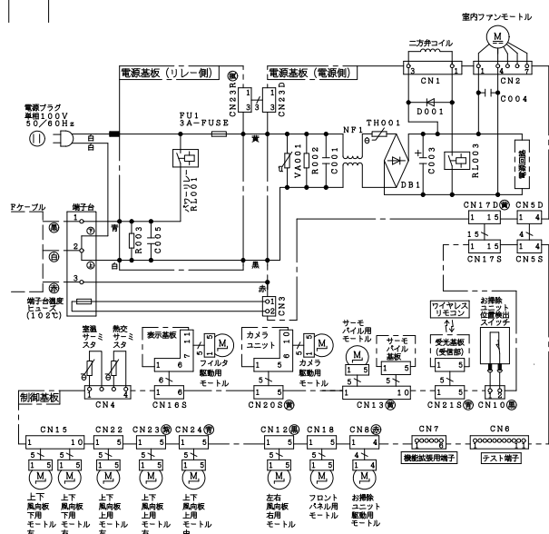
配線図 RAS-ZJ25G
