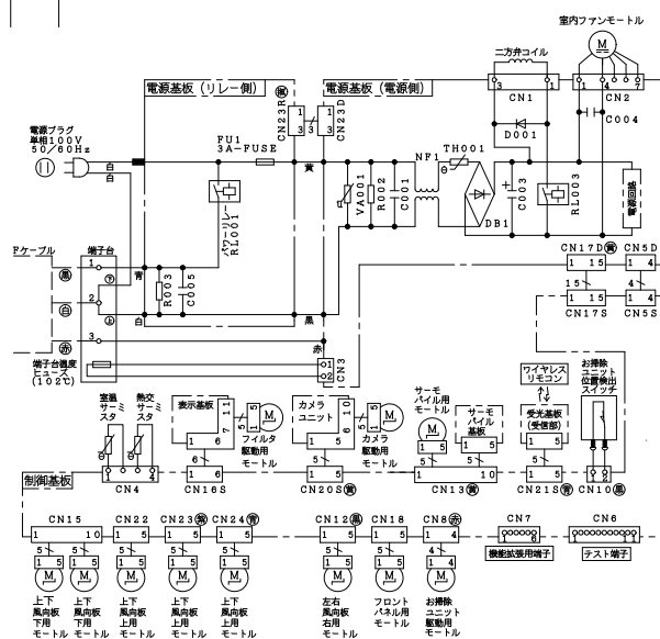
配線図 RAS-ZJ22G
