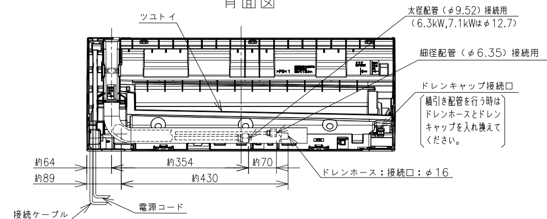
背面図
