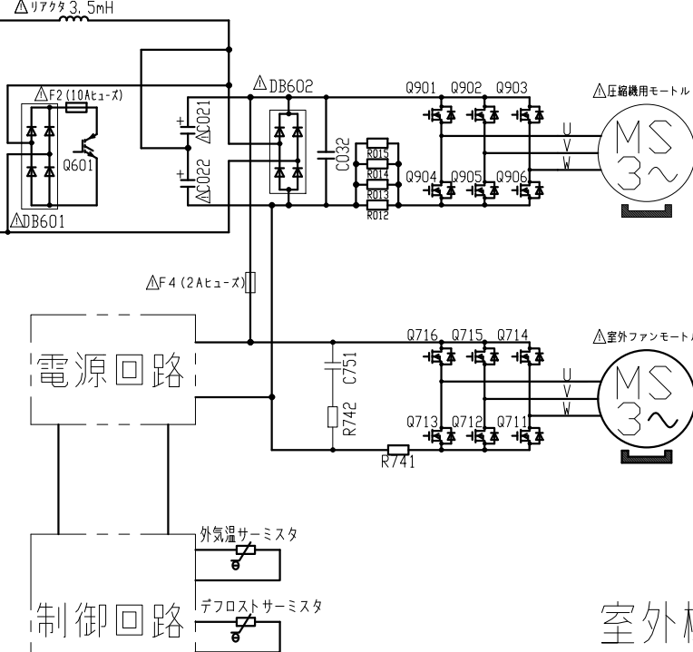
室外機配線図
