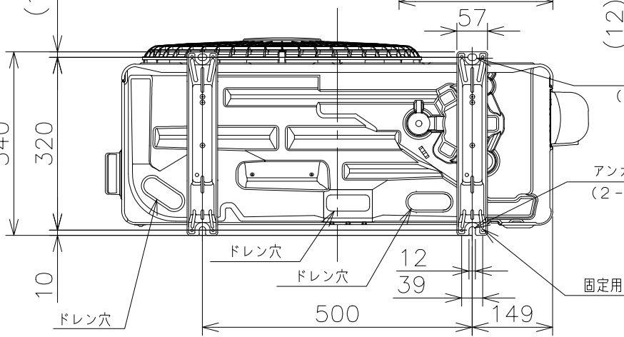
背面図
