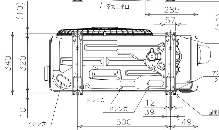
背面図
