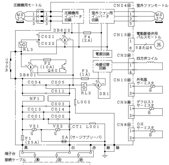
配線図 R A C - X J 2 2 F
