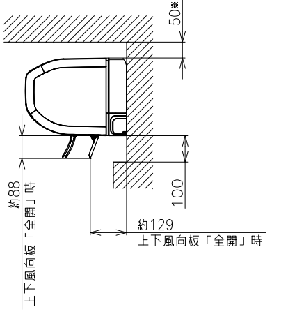
※室内機の背面で配管接続する 場合は110mm以上
