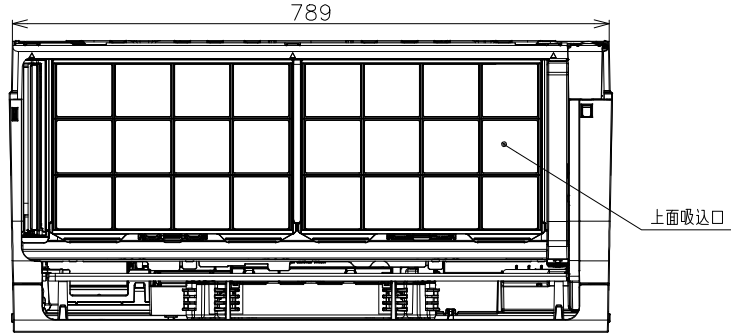
日立ルームエアコン壁掛XCシリーズ 室内ユニット寸法図
