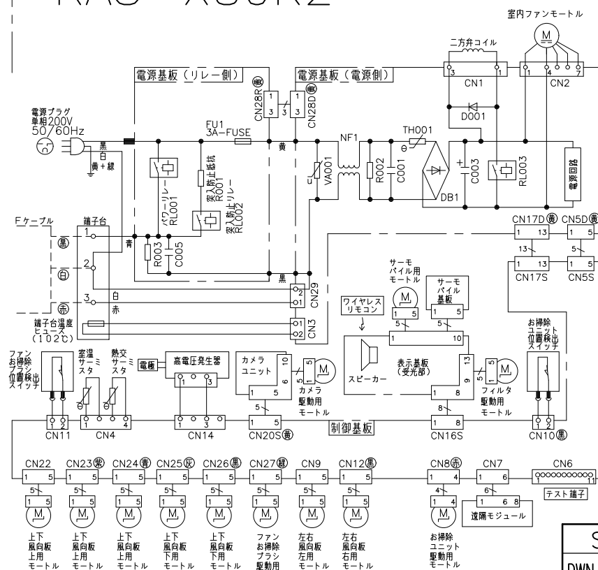
配線図 RAS-X80K2
