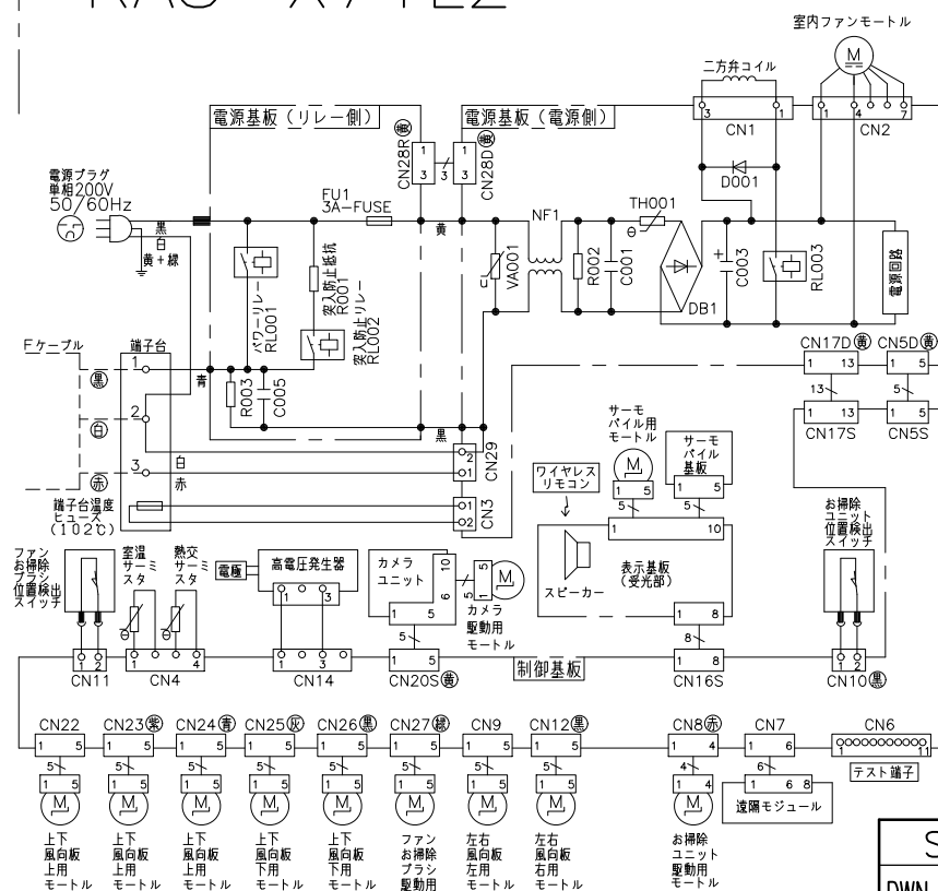
配線図 RAS-X71L2
