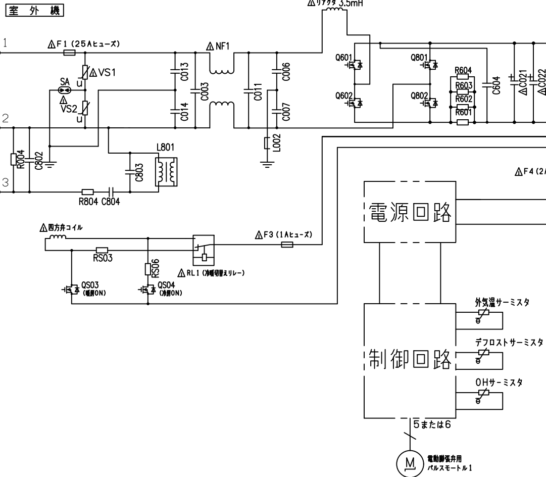
配線図 RAS-X71L2
