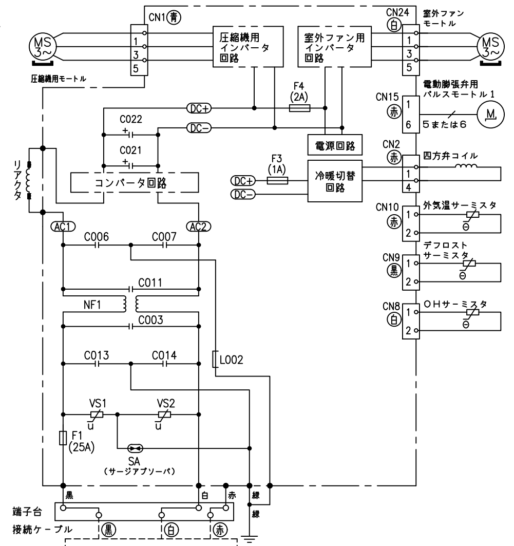
配線図 RAC-X71L2
