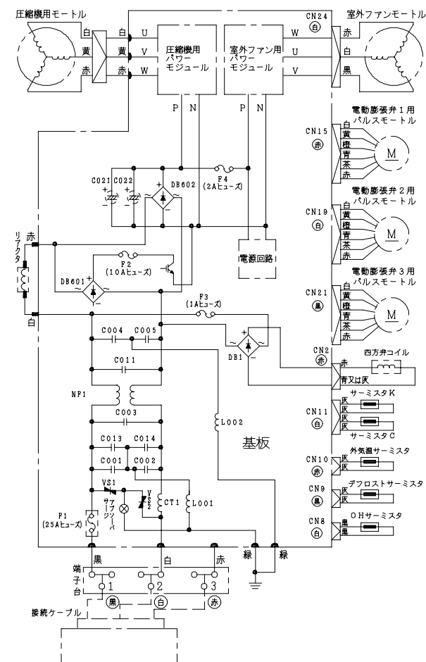
配線図 R A C - X 5 0 W 2
