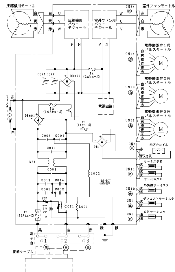
配線図 R A C - X 4 0 W 2
