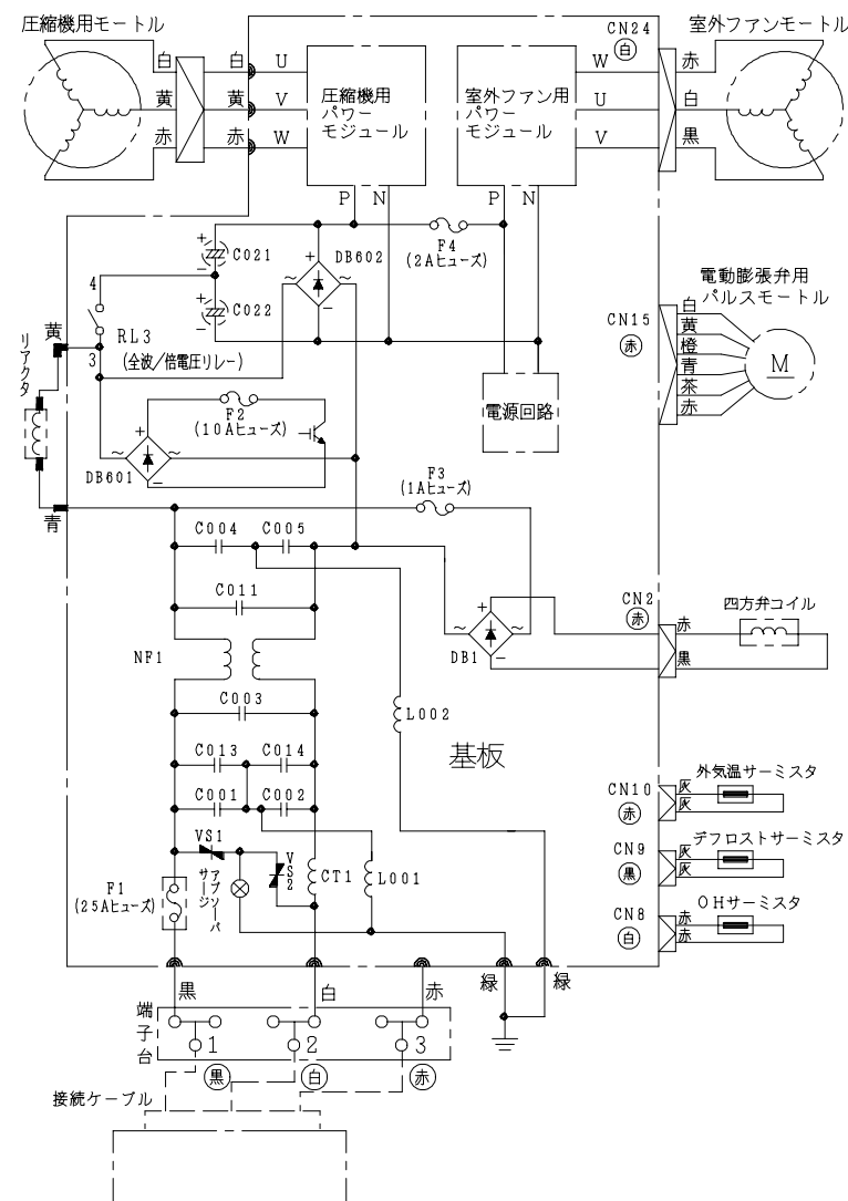
配線図 RAC-X36X
