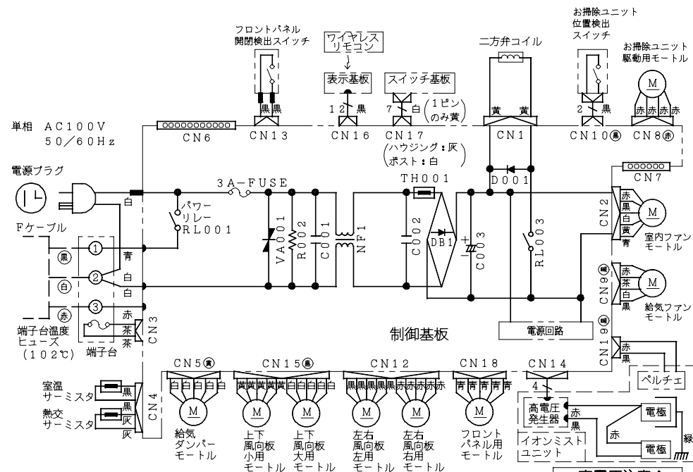
配線図 RAS-X36X
