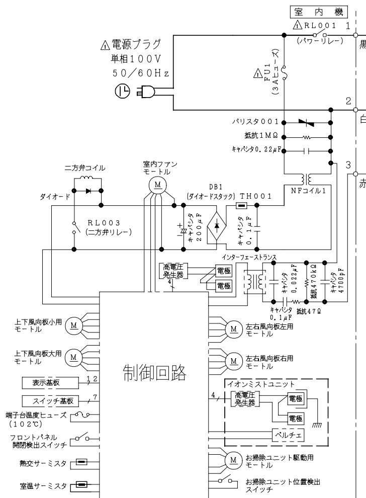
回路図
