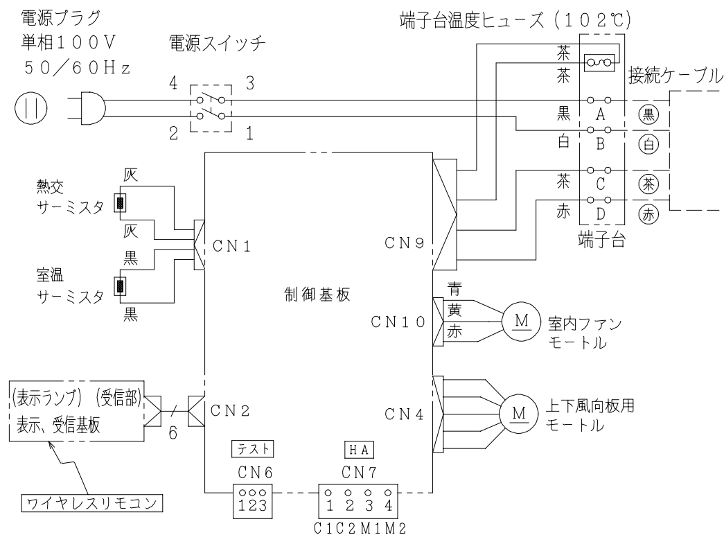
配線図 RAS-X25JX
