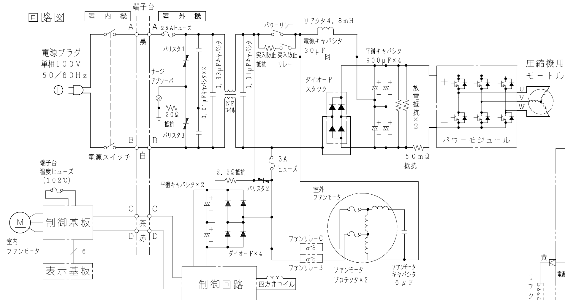
配線図 RAS-X25JX
