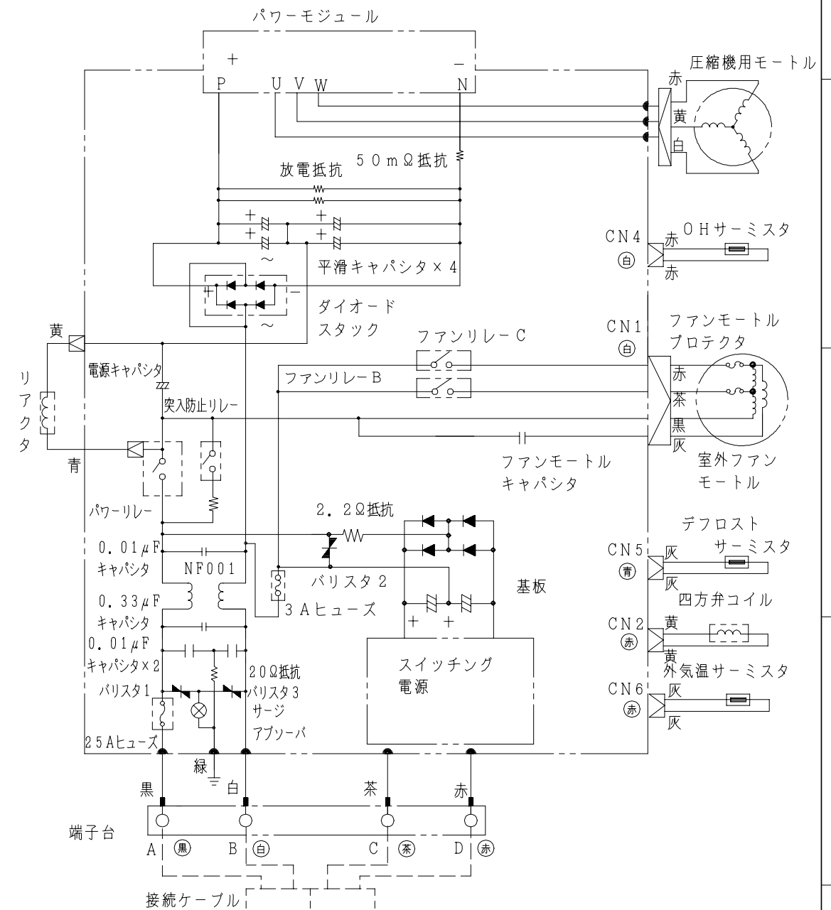
配線図 RAC-258JX
