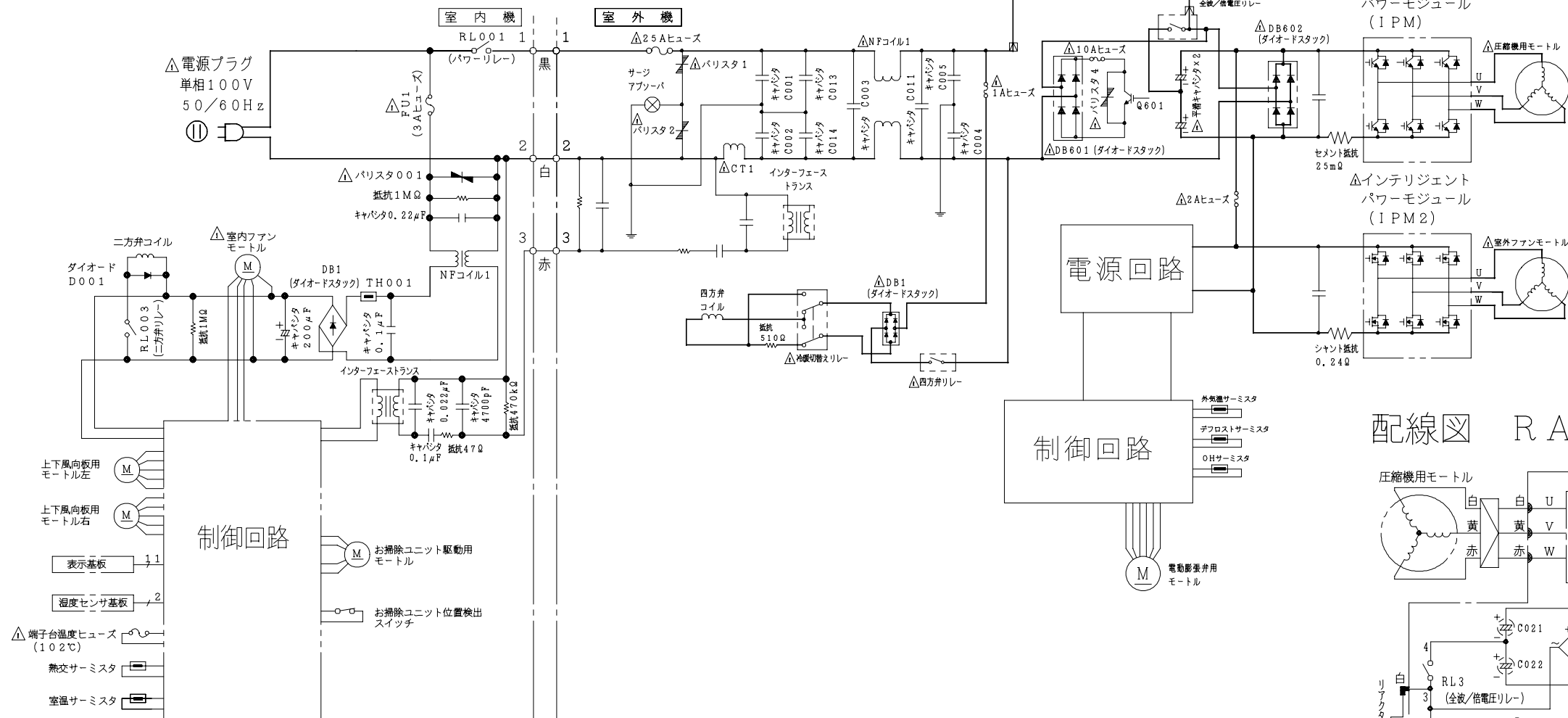
配線図 RAS-VJ36A
