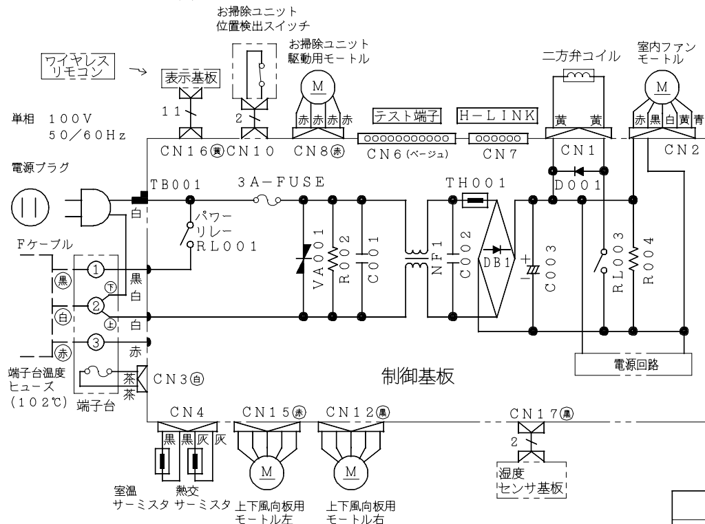
配線図 RAS-VJ36A
