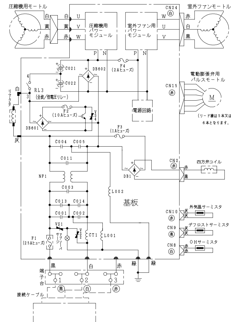
配線図 RAC-VJ36A
