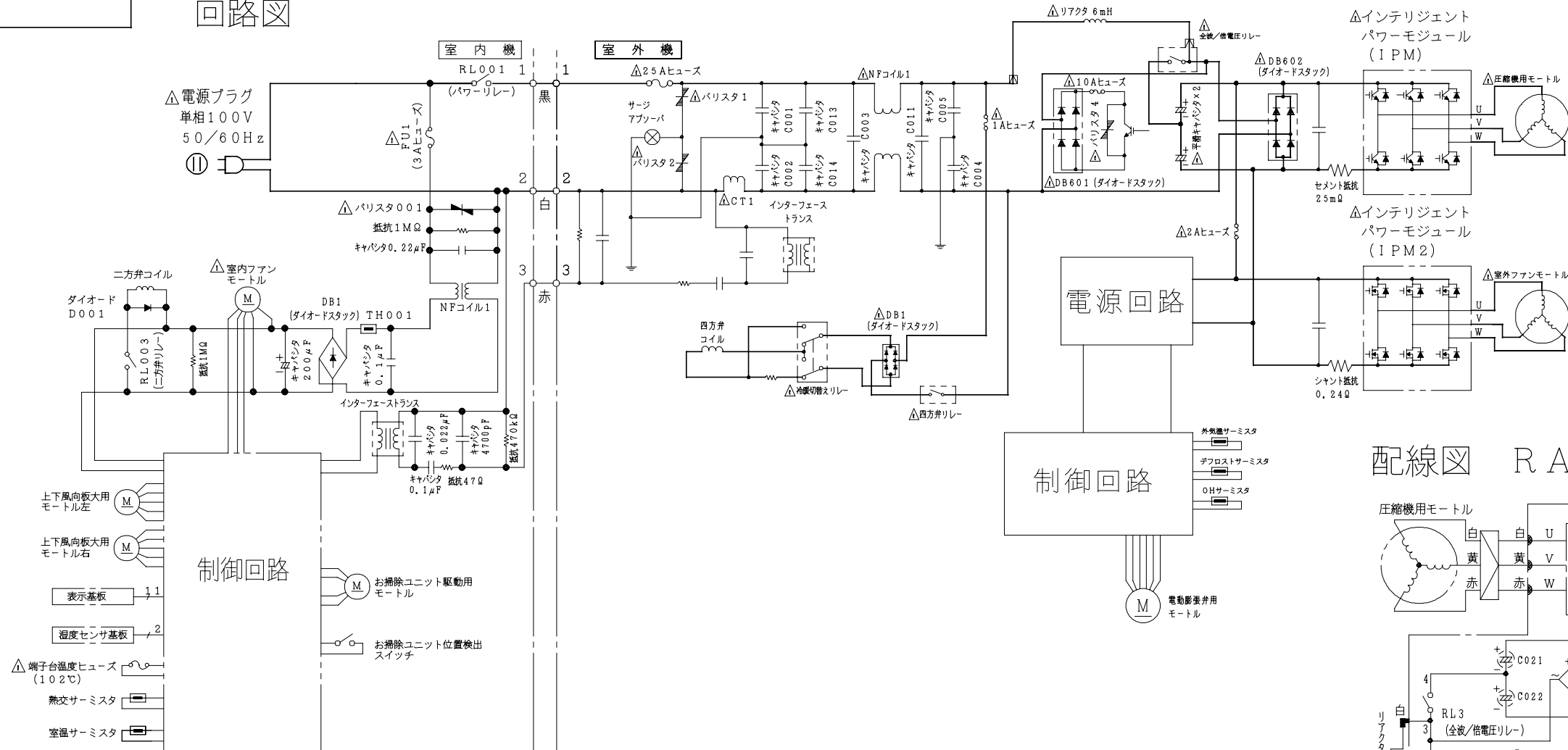
配線図 RAS-VJ25Z
