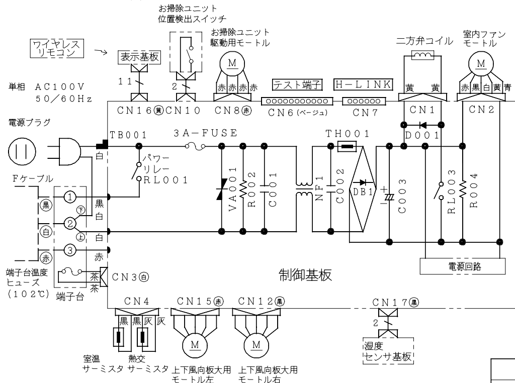
配線図 RAS-VJ25Z
