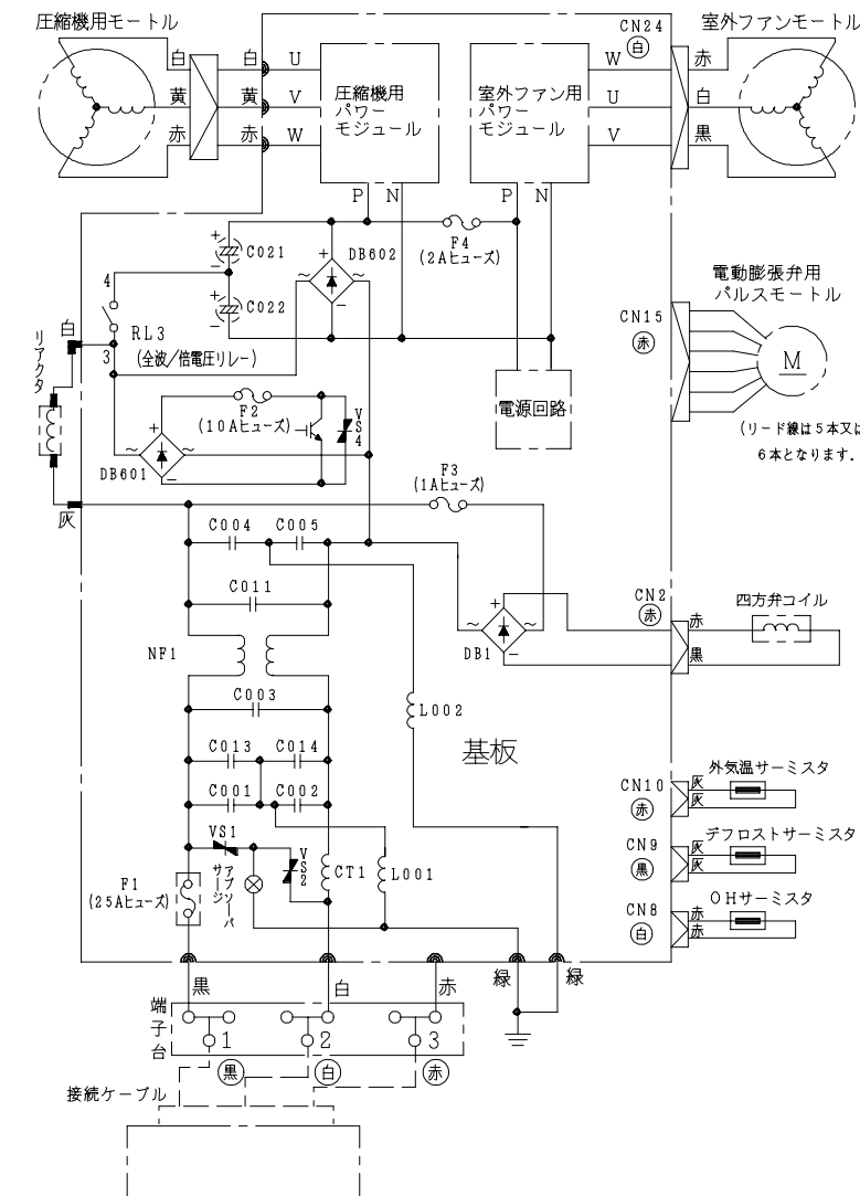
配線図 RAC-VJ25Z
