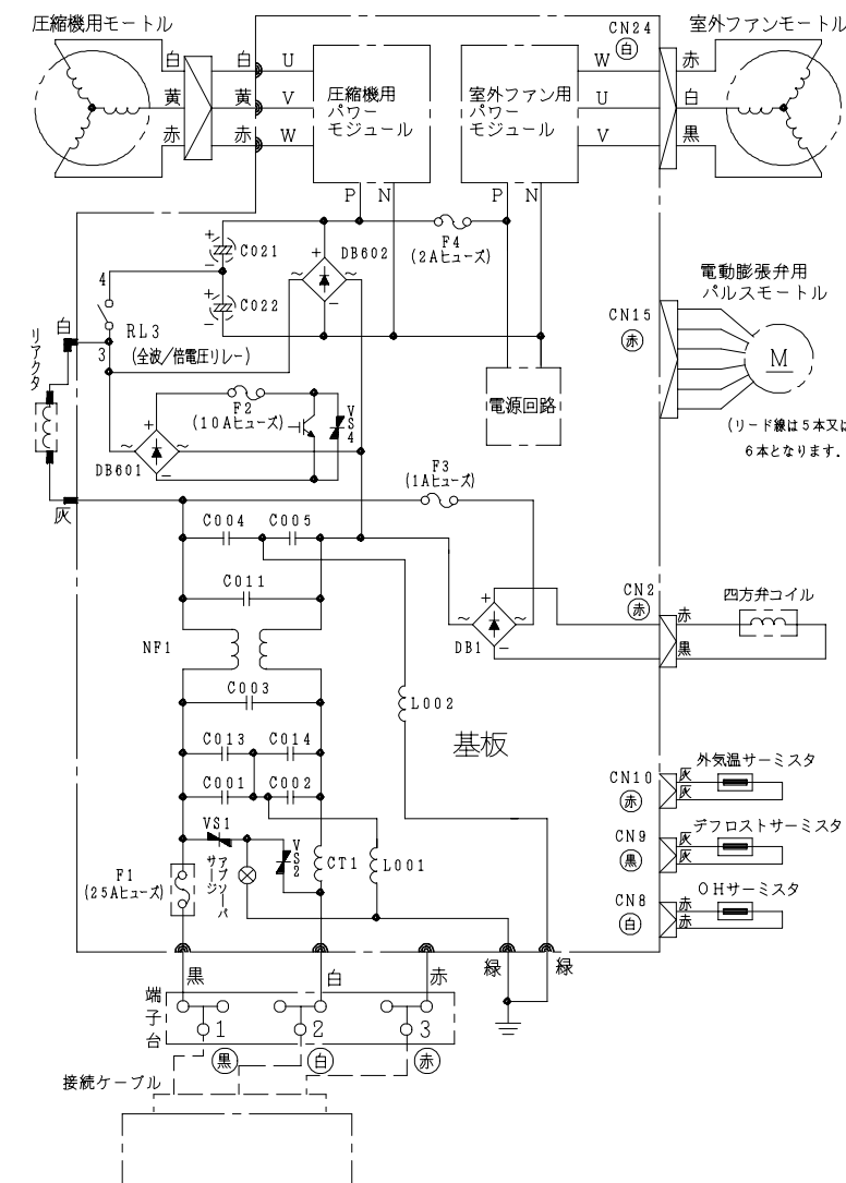
配線図 RAC-VJ25A
