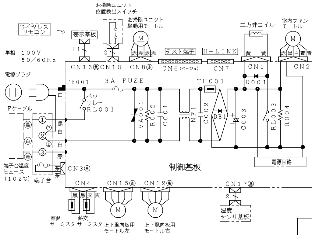
配線図 RAS-VJ25A
