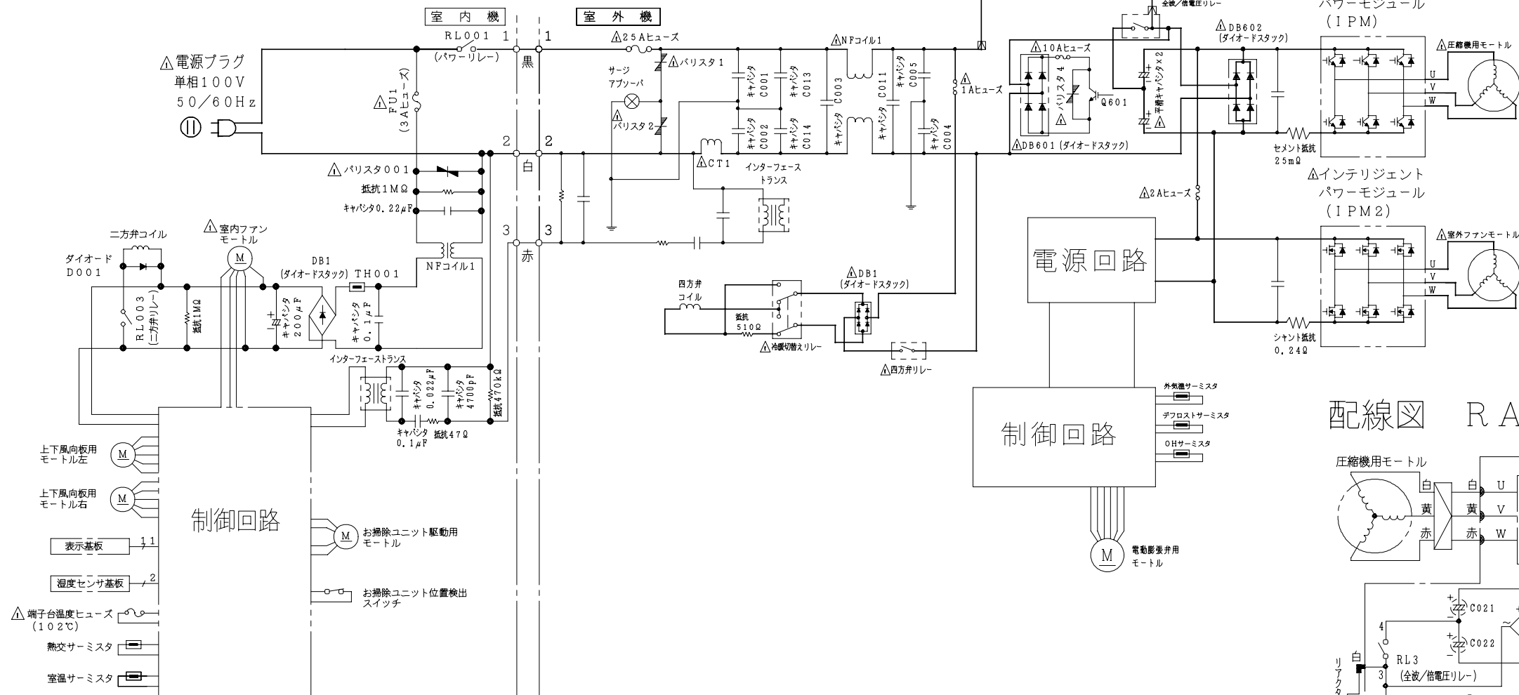
配線図 RAS-VJ25A
