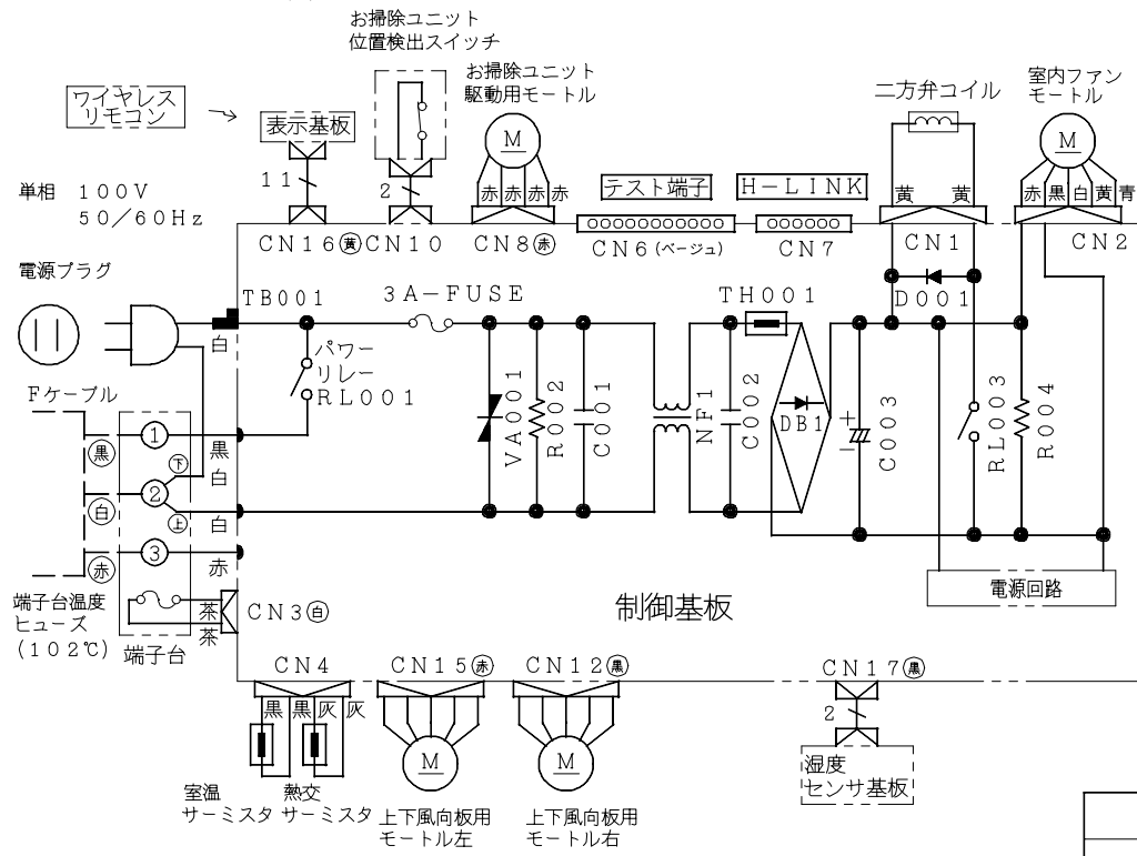
配線図 RAS-VJ22A
