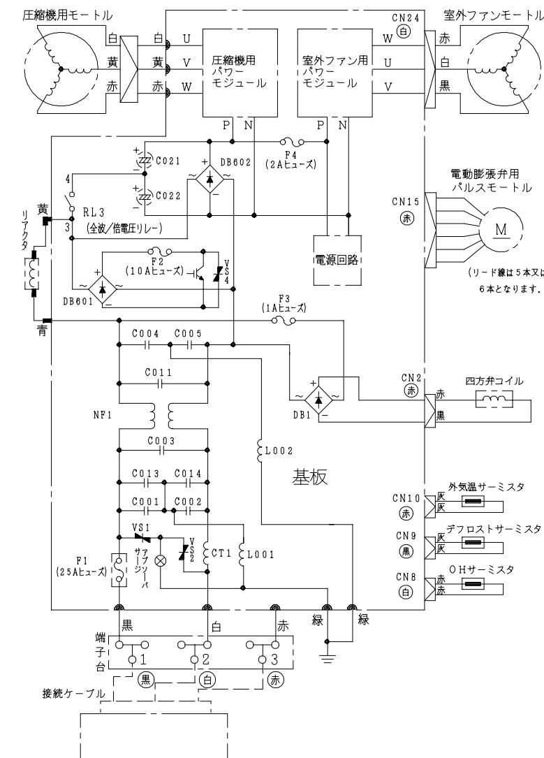
配線図 RAC-VJ22A
