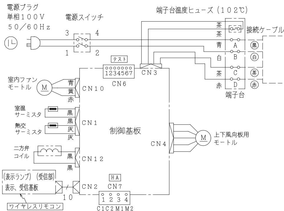
配線図 R A S - V 3 2 K X
