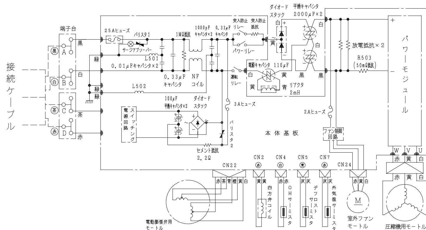
配線図 R A C - 3 2 K X
