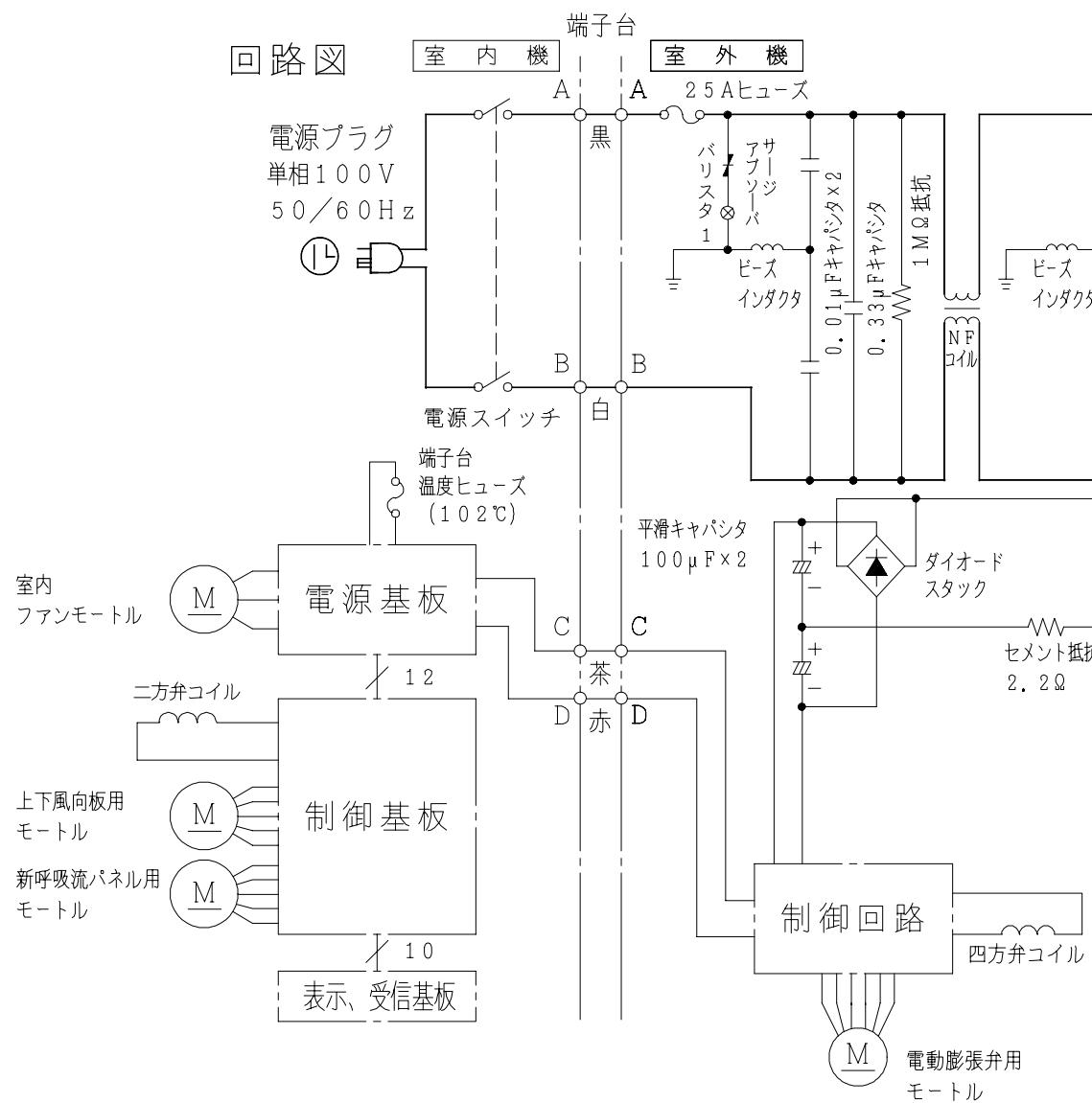
配線図 RAS-V32JX
