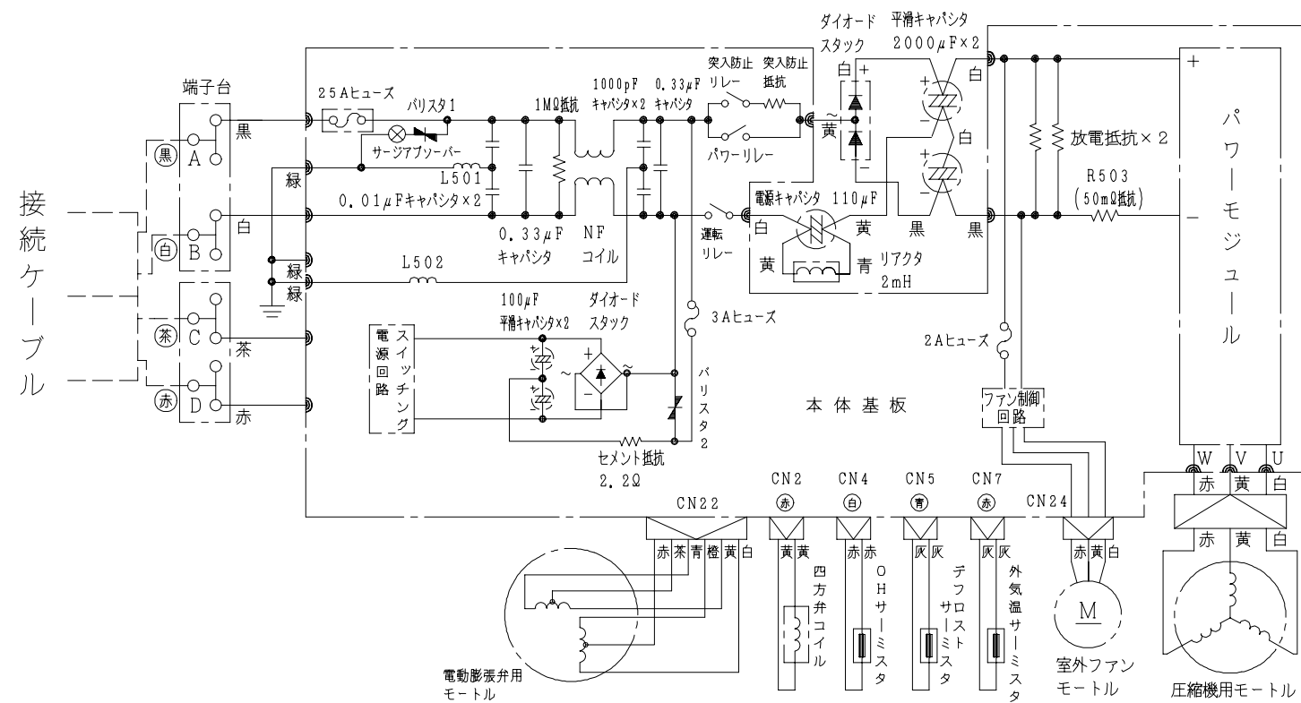
配線図 RAC-329JX
