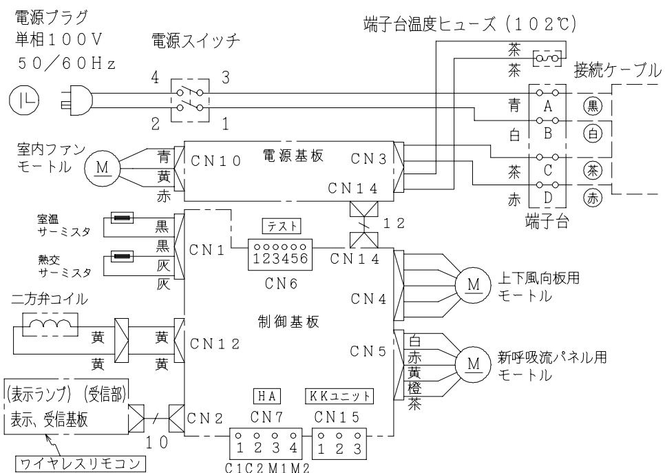
配線図 RAS-V32JX
