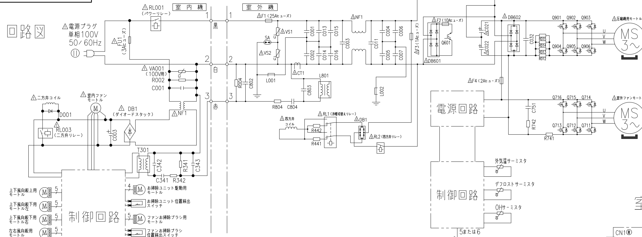
室内機配線図
