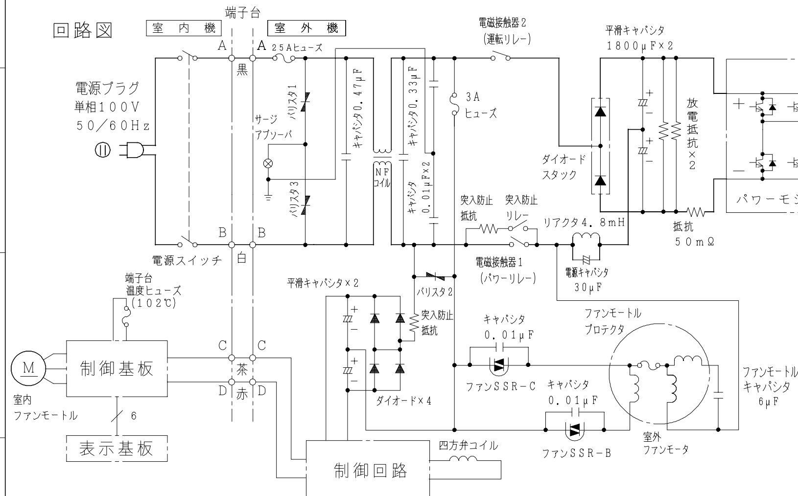
配線図 RAS-V25KX
