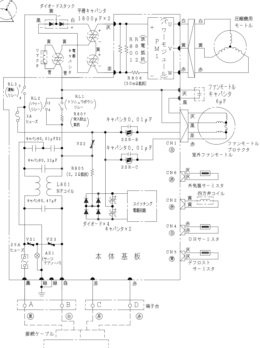
配線図 RAC-258KX
