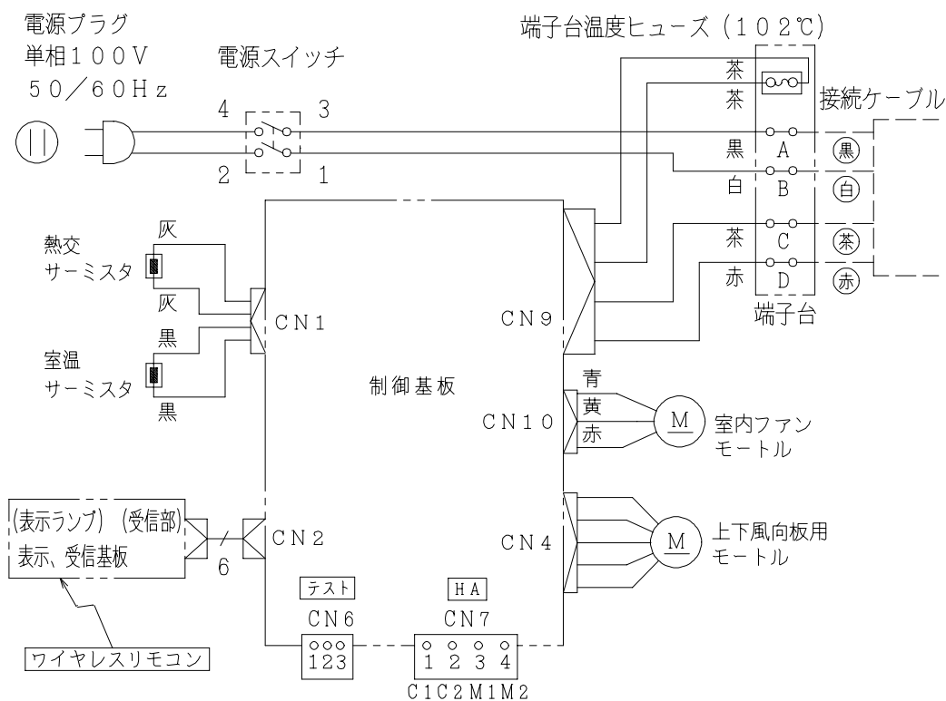
配線図 RAS-V25KX
