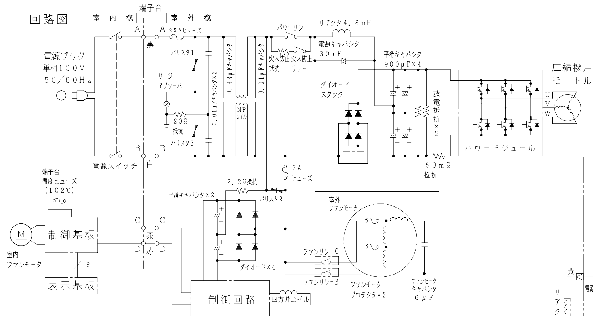
配線図 RAS-V25JX
