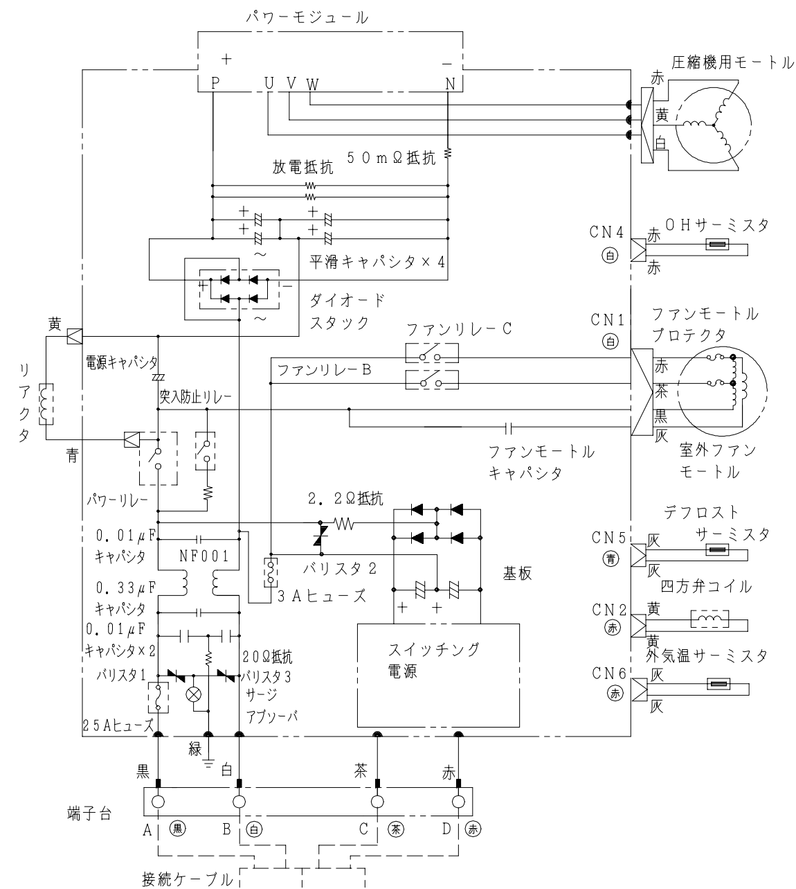
配線図 RAC-258JX
