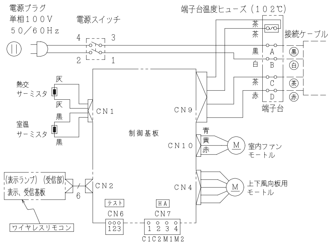
配線図 RAS-V25JX
