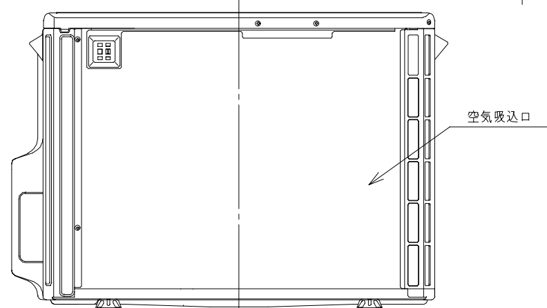
背面図
