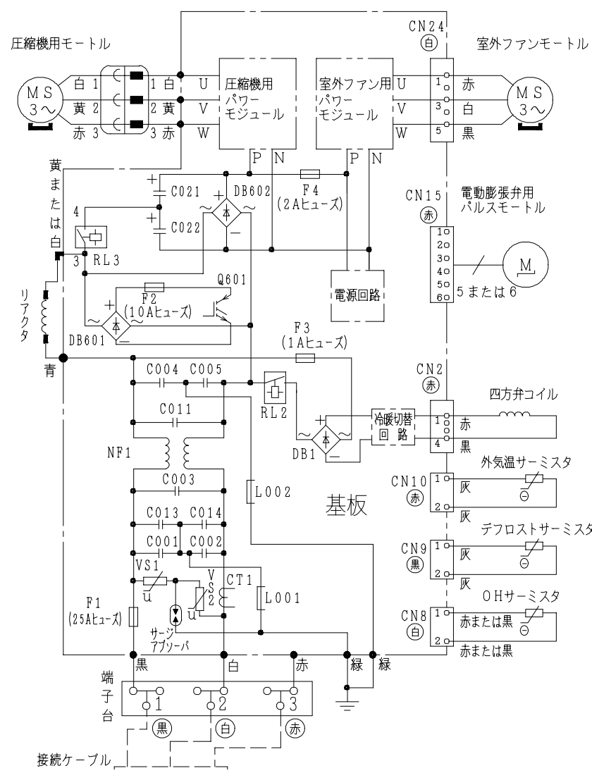
配線図 RAC-SN22C
