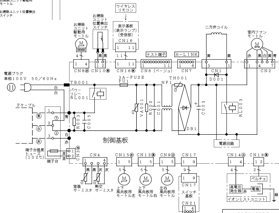
配線図 RAS-SN22C
