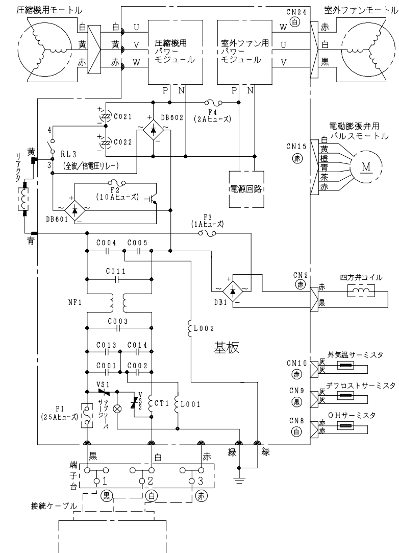
配線図 RAC-SC36X
