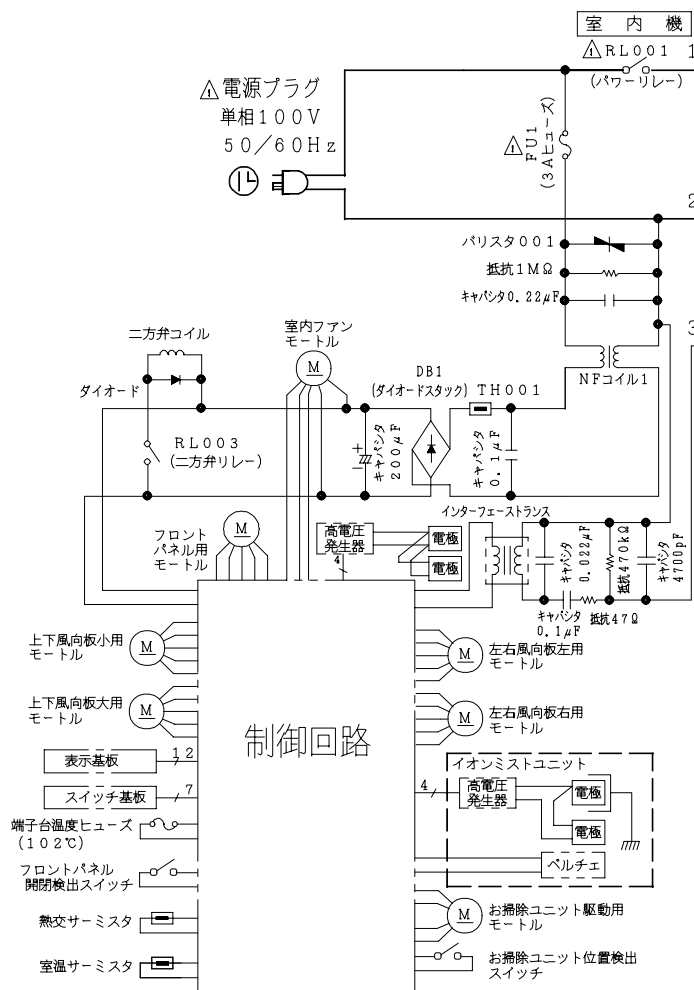
回路図
