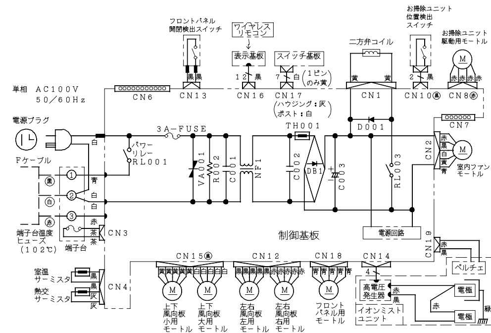
配線図 RAS-SC36X
