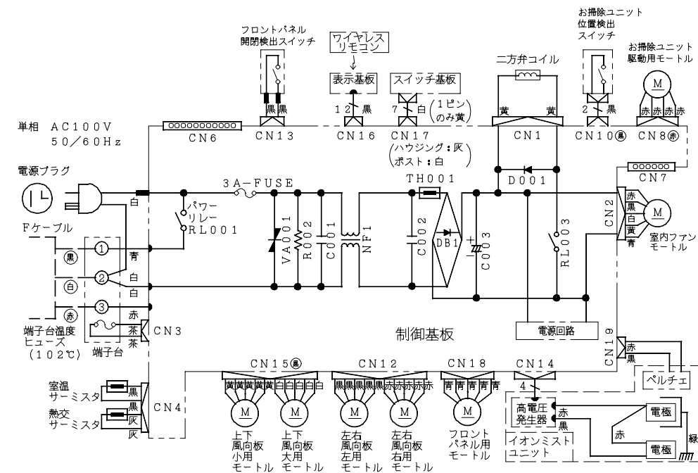
配線図 RAS-S36X
