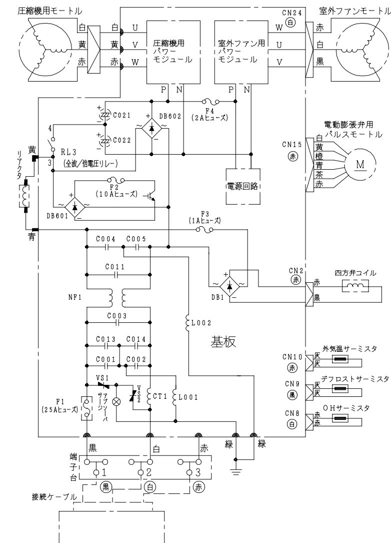
配線図 RAC-S36X
