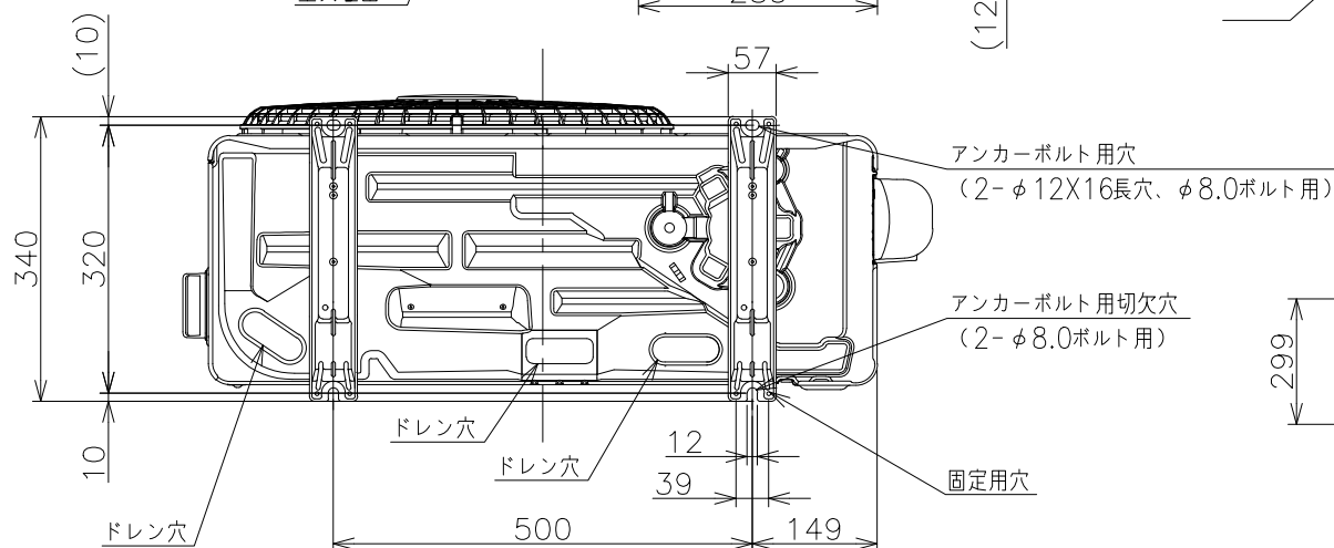
背面図
