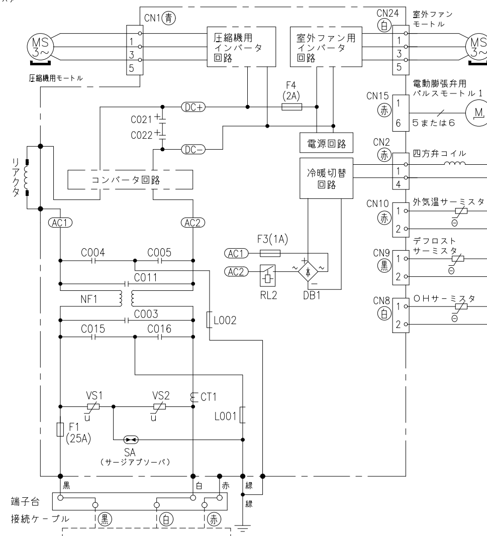
配線図 RAC-S36K
