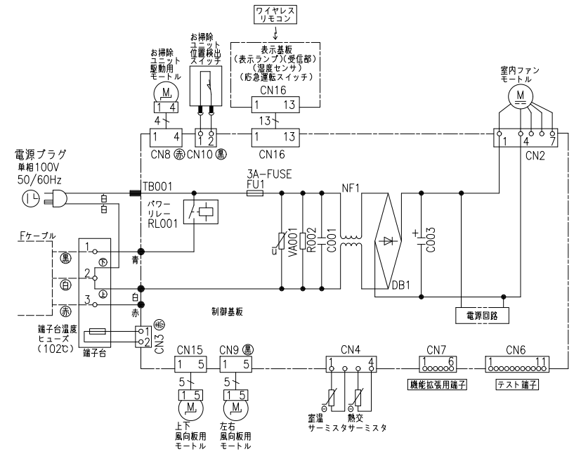
室内機配線図
