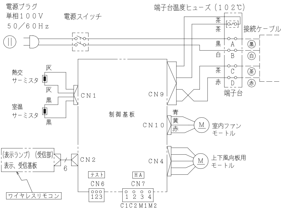
配線図 RAS-R22NX
