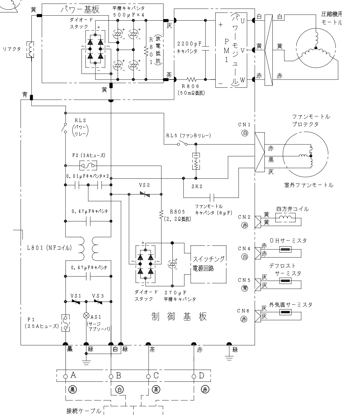
配線図 RAC-22NX
