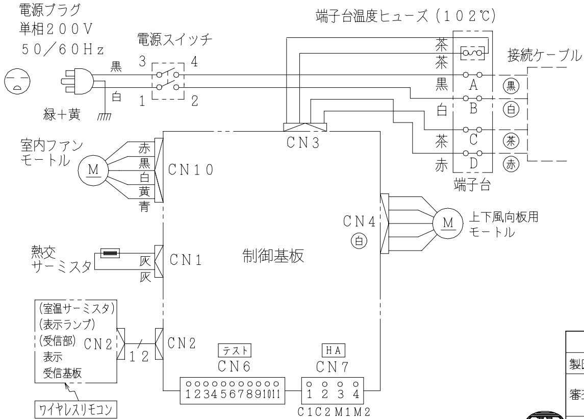
配線図 RAS-N40T2
