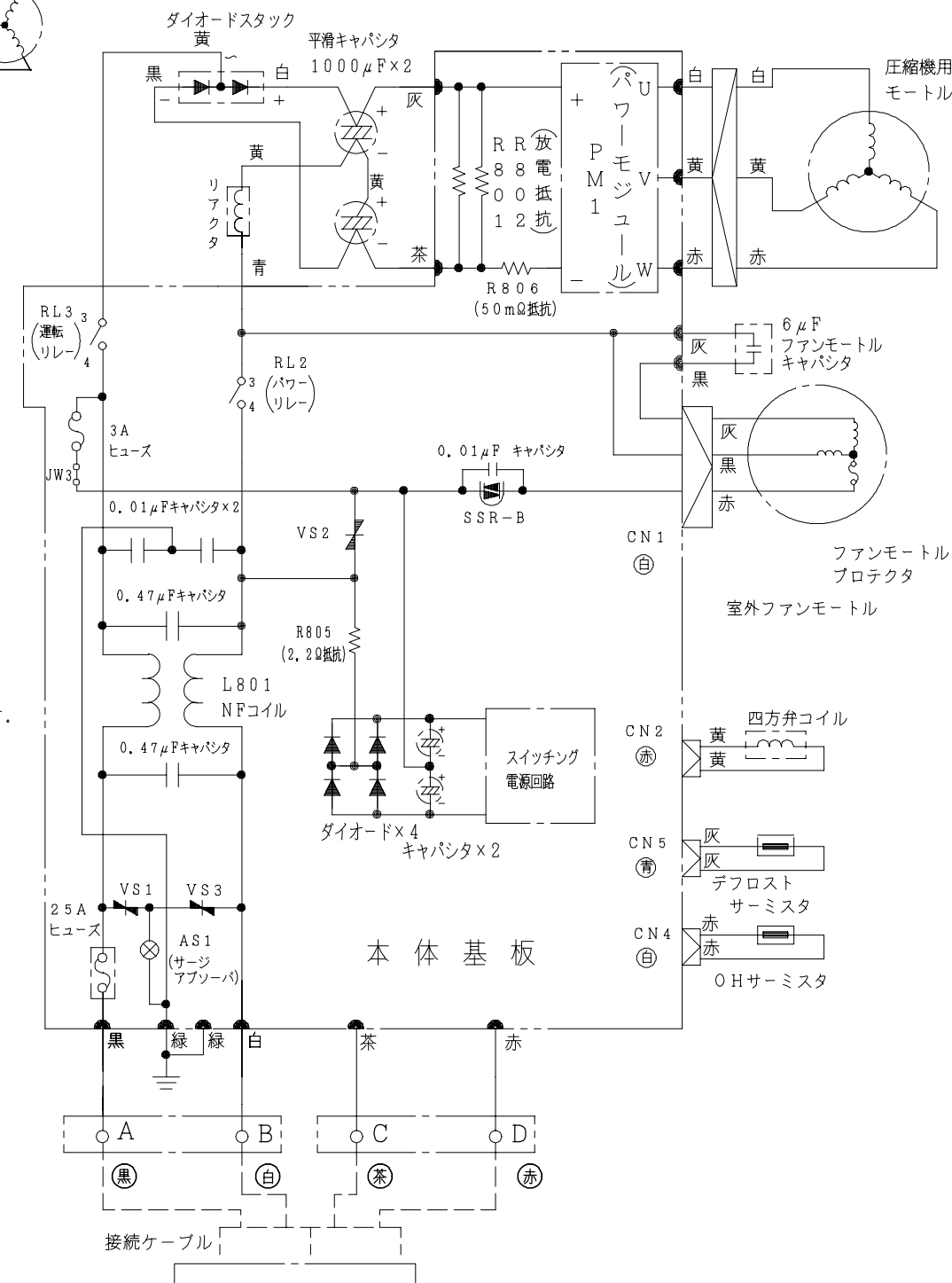
配線図 RAC-22GX
