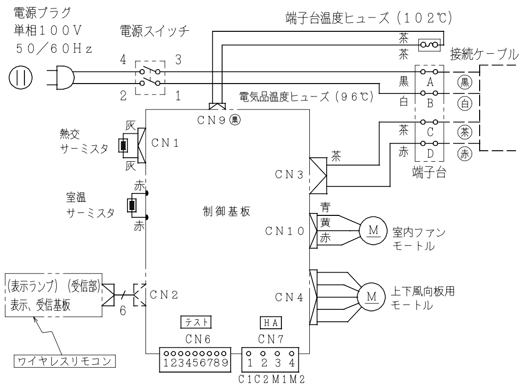
配線図 RAS-N22GX
