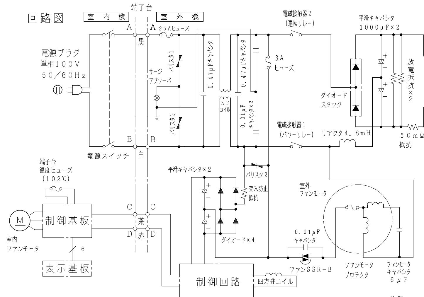
配線図 RAS-N22GX
