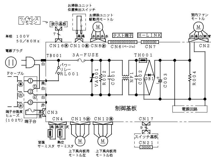
配線図 R A S - M Z 2 2 A
