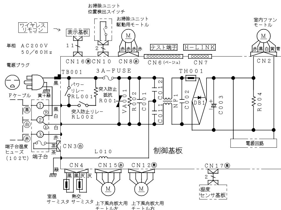
配線図 R A S - M 4 0 Z 2
