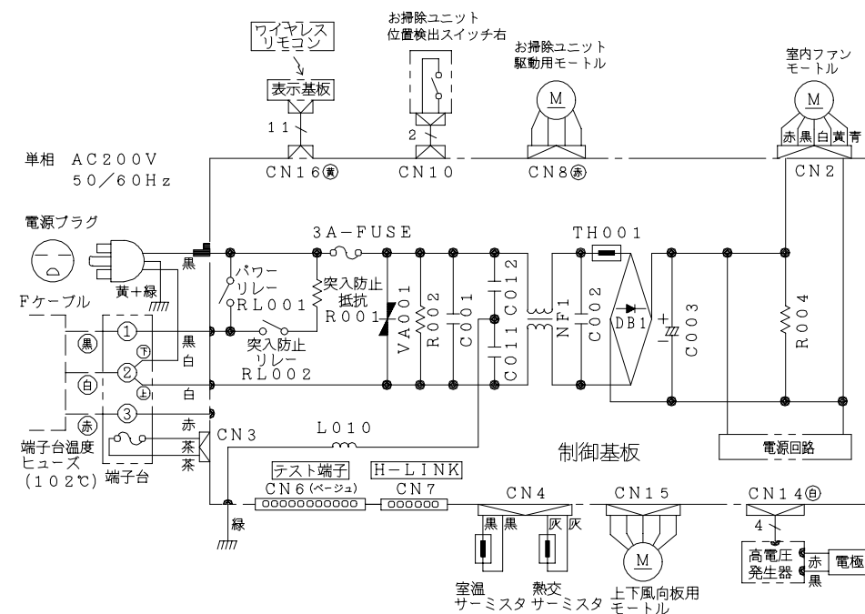
配線図 RAS-M40X2
