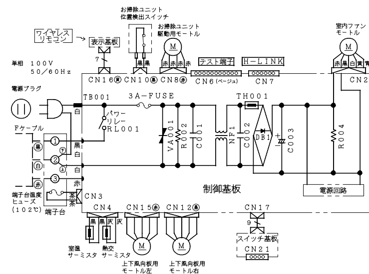
配線図 R A S - M 3 6 A
