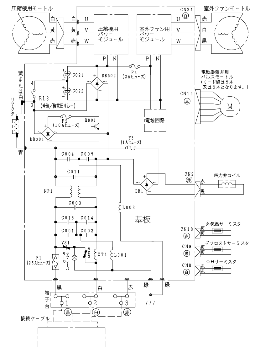
配線図 R A C - M 3 6 A
