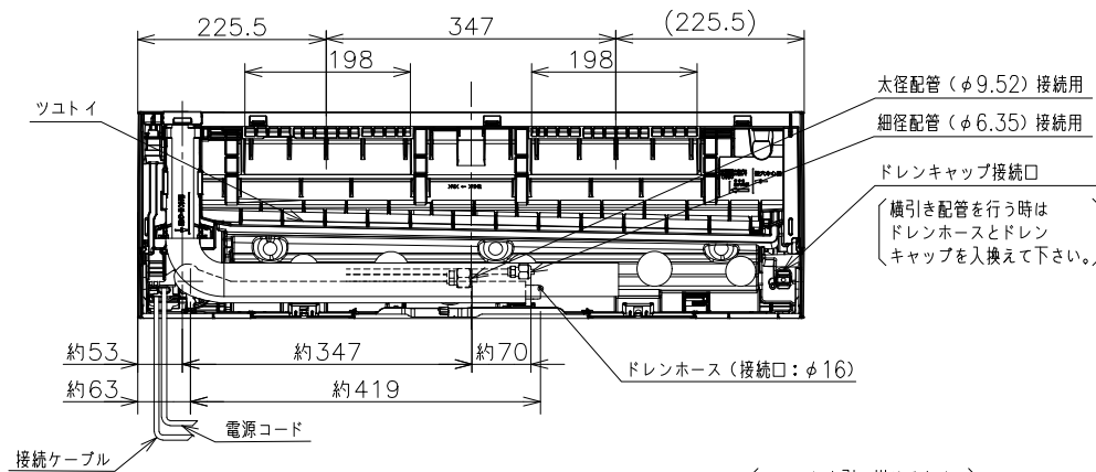
背面図
