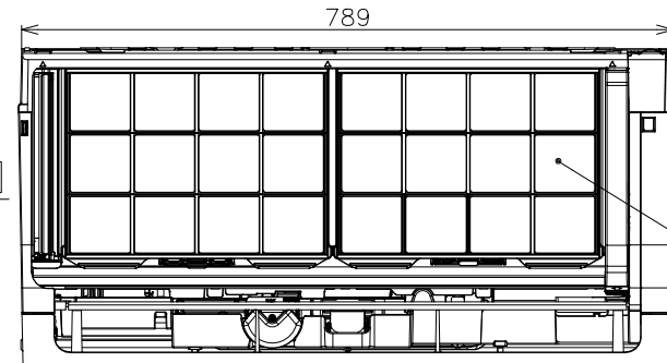
日立ルームエアコン 壁掛KSシリーズ室内ユニット 寸法図
