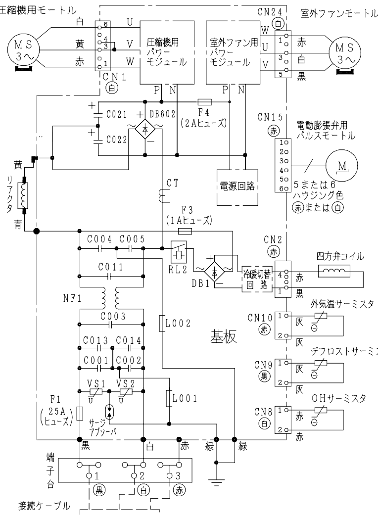
配線図 RAC-KJ22C
