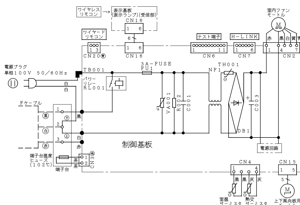
配線図 RAS-KJ22C
