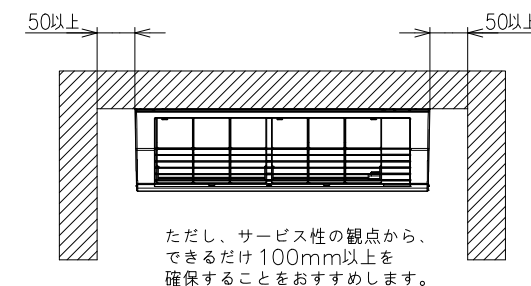
室内機サービススペース
