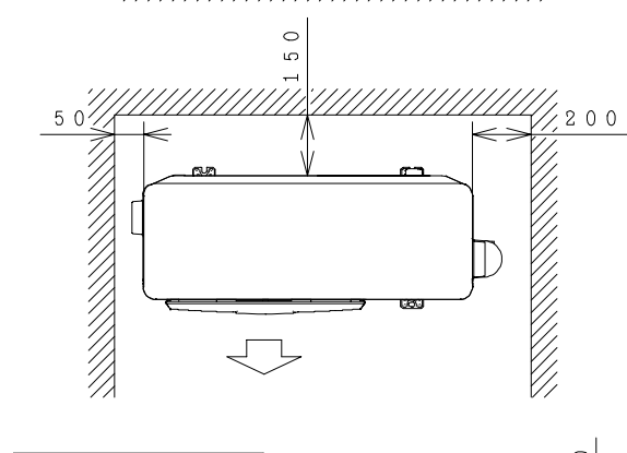
前後のみに壁がある場合
