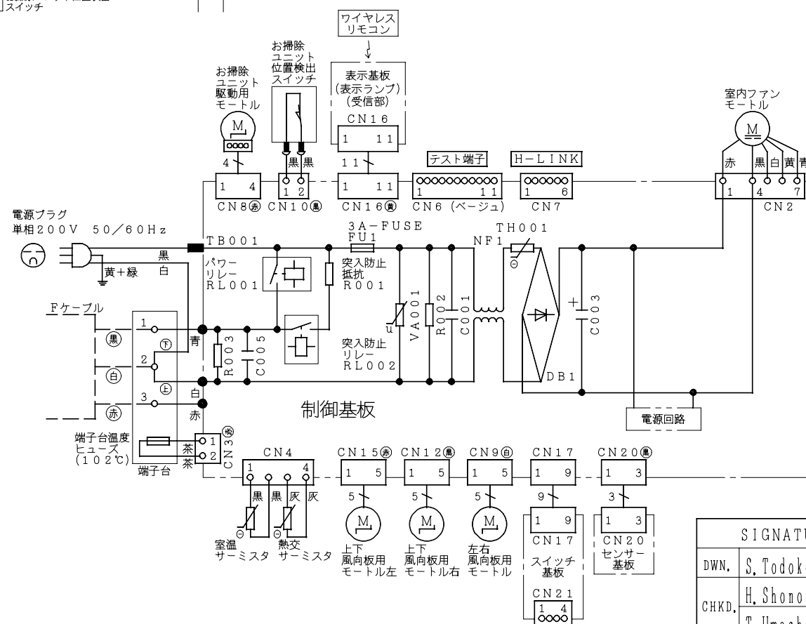
配線図 R A S - K 4 0 B 2
