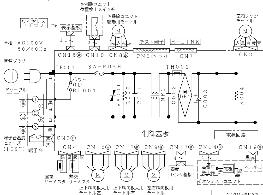
配線図 RAS-K22Z
