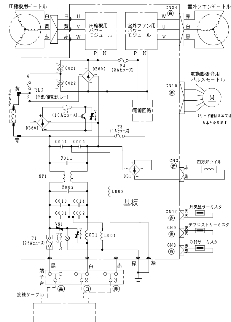
配線図 RAC-K22Z
