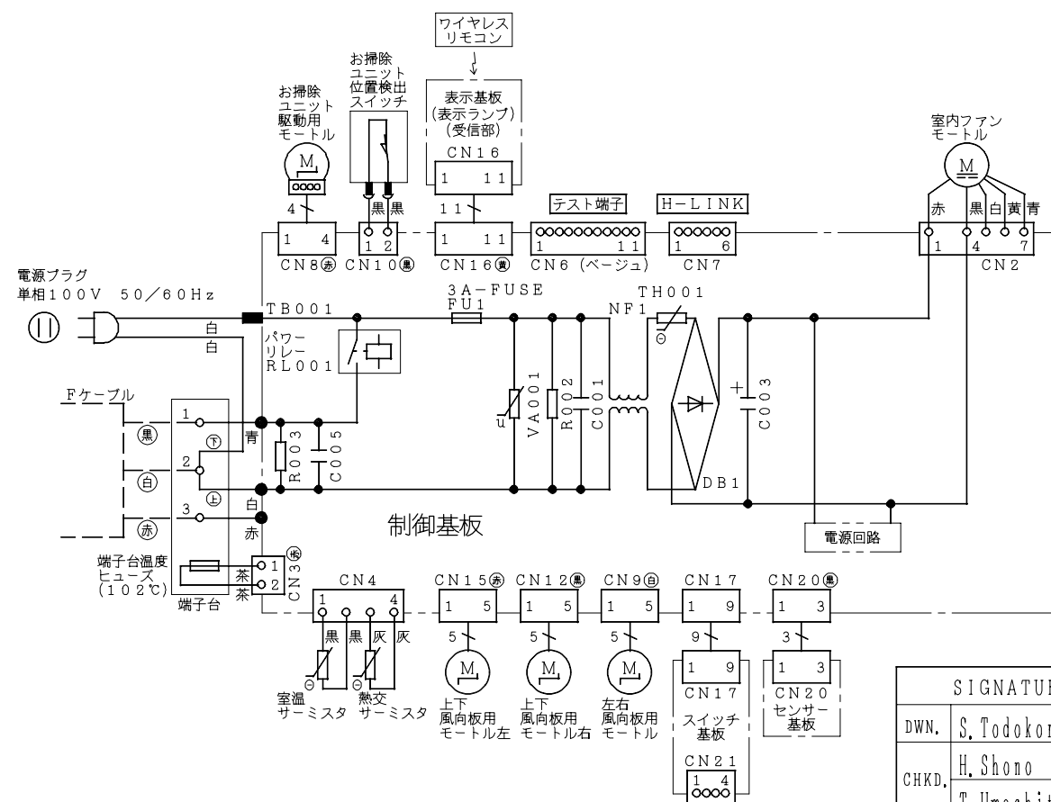
配線図 RAS-K22B
