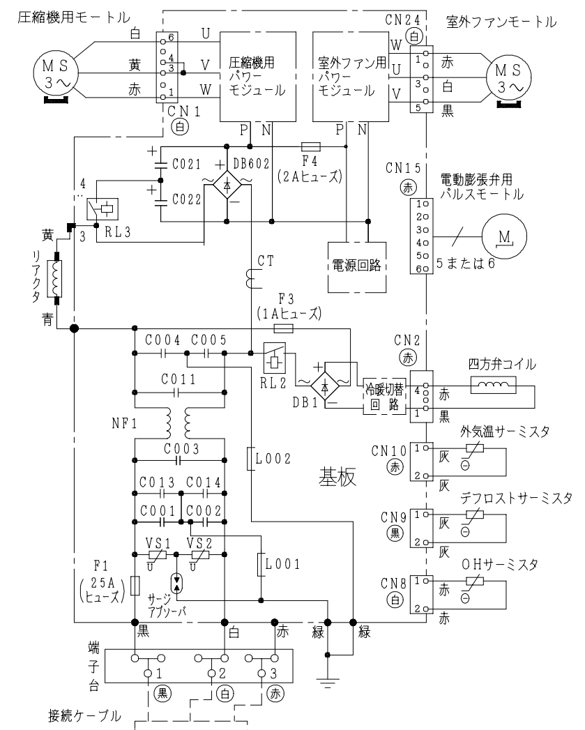
配線図 RAC-K22B
