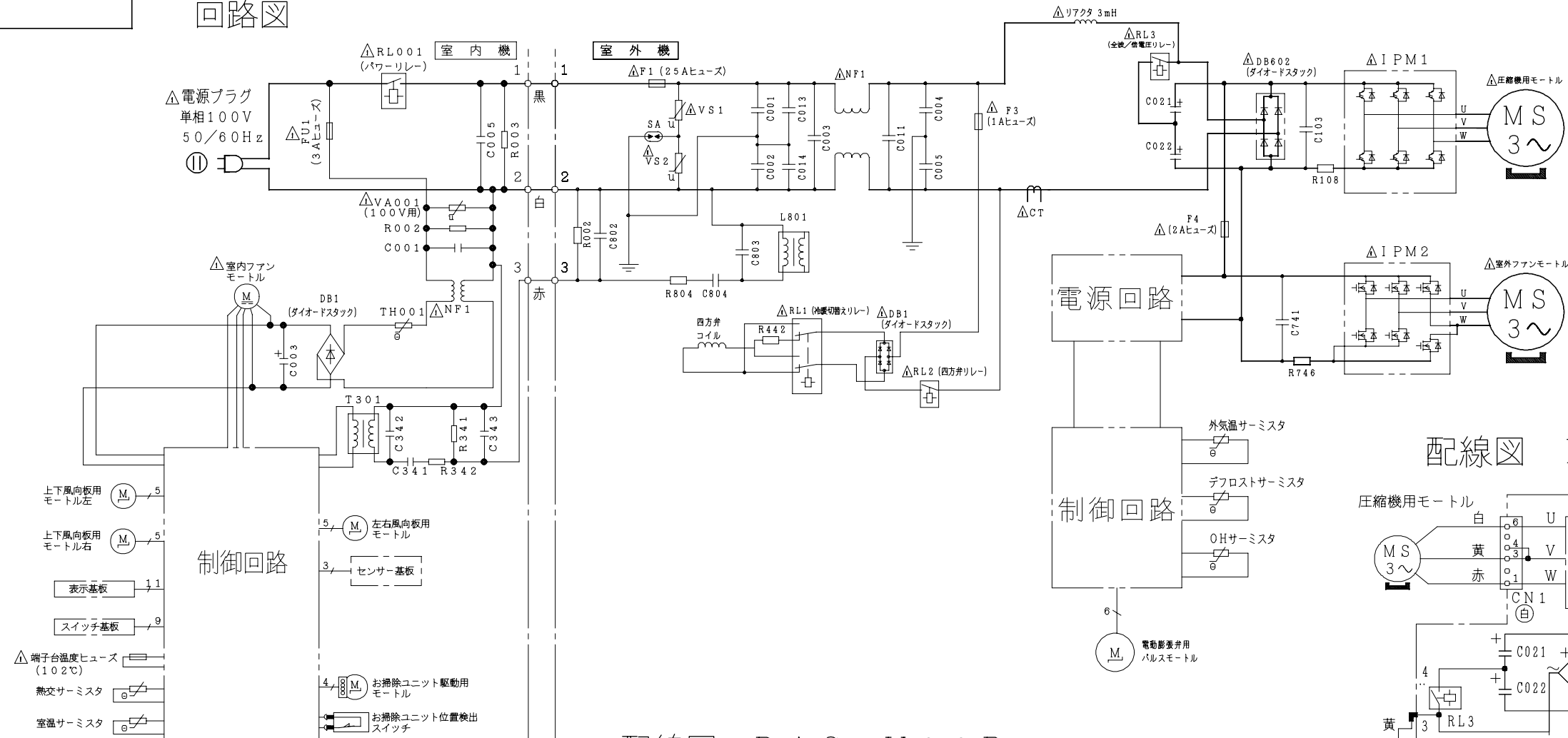
配線図 RAS-K22B
