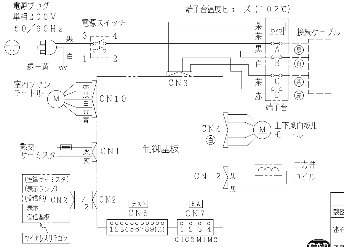
配線図 RAC-G40V2
