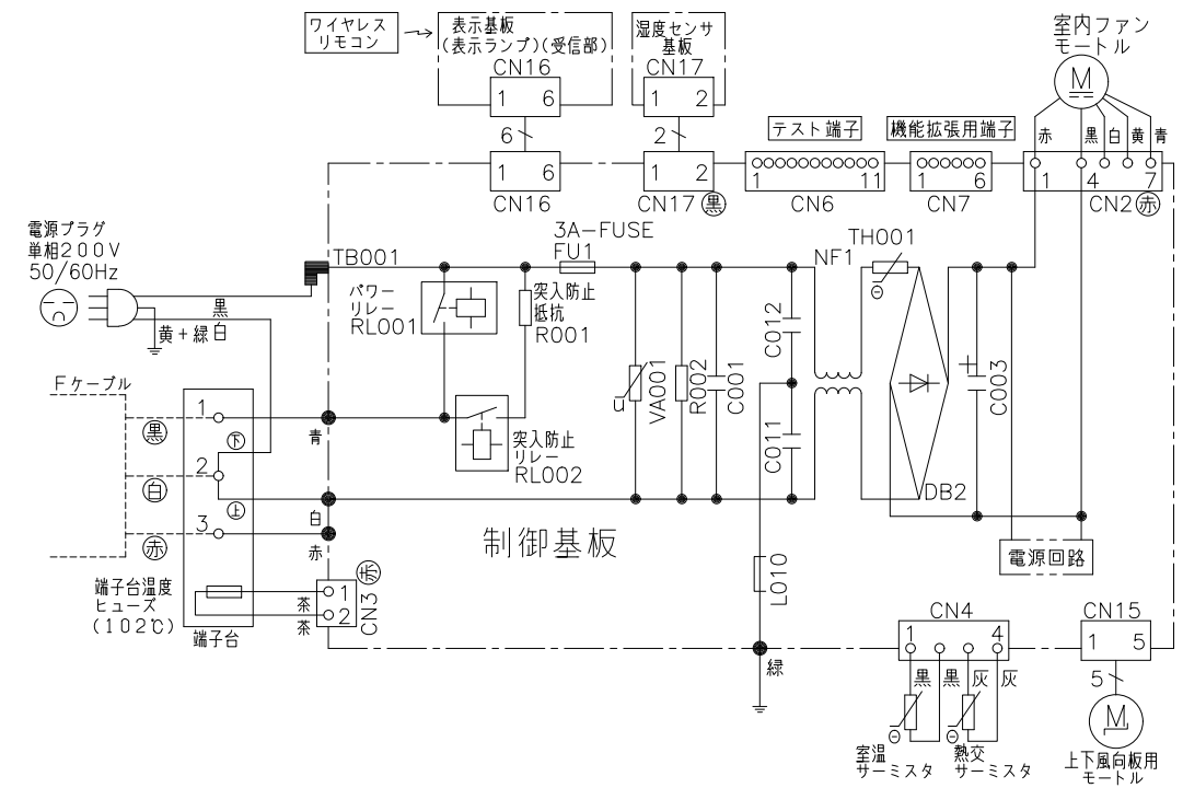
配線図 RAS-F40J2
