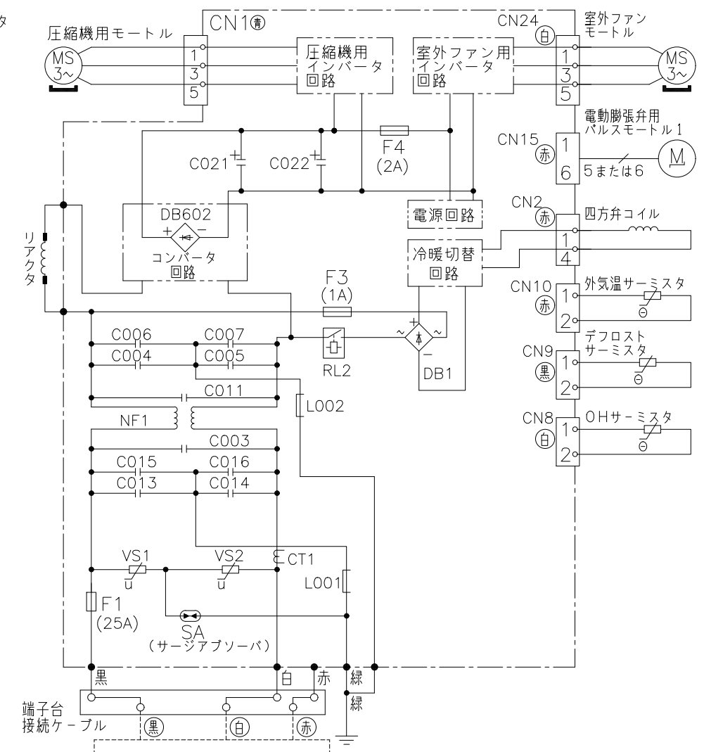
配線図 RAC-F40J2
